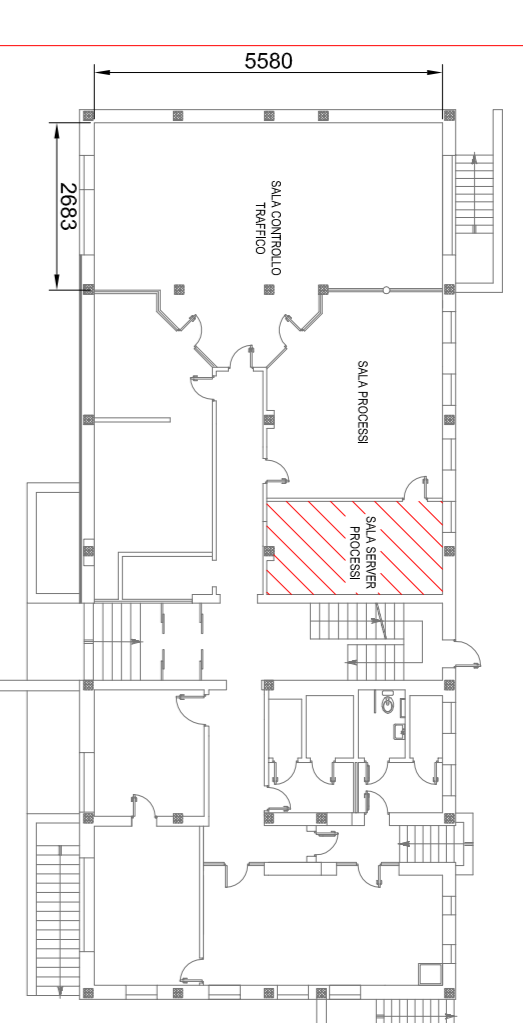
PIANO PRIMO - PALAZZINA ESERCIZIO PRESSO SEDE CAV
