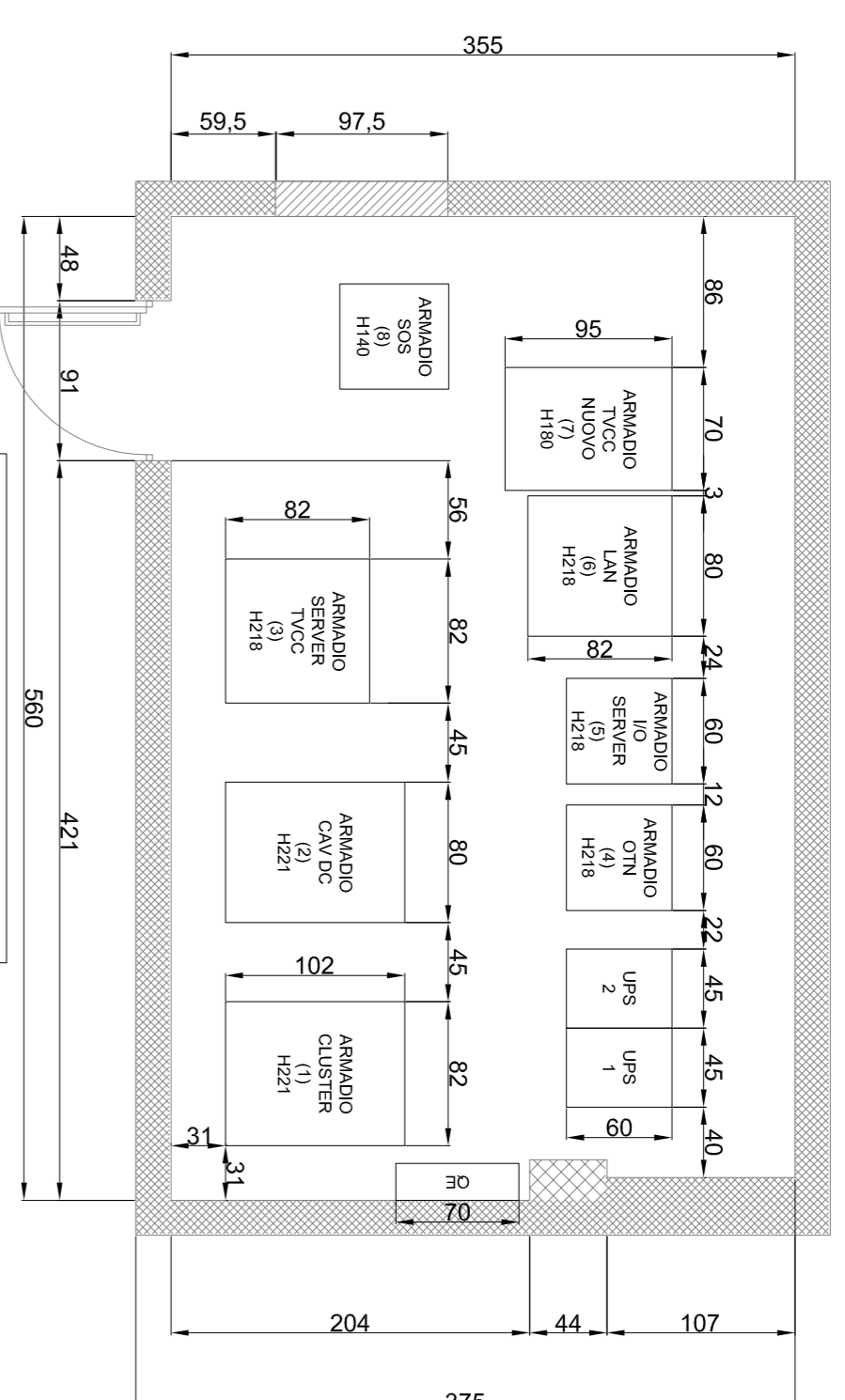
DISPOSIZIONE APPARECCHIATURE Sala Server Processi
