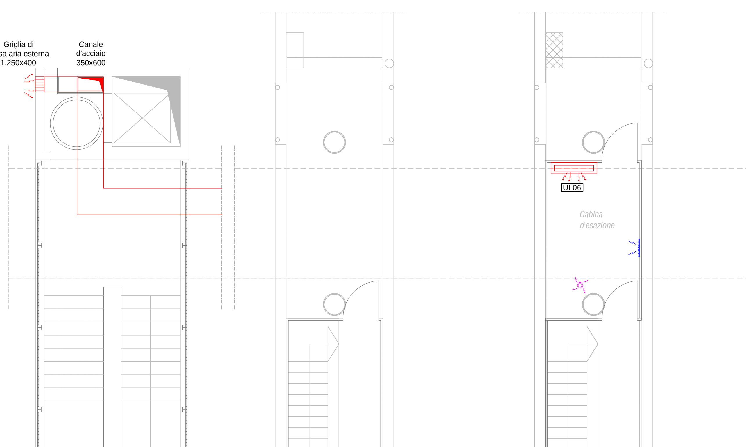
Pianta piano terra - cabine di esazione scala 1:50
