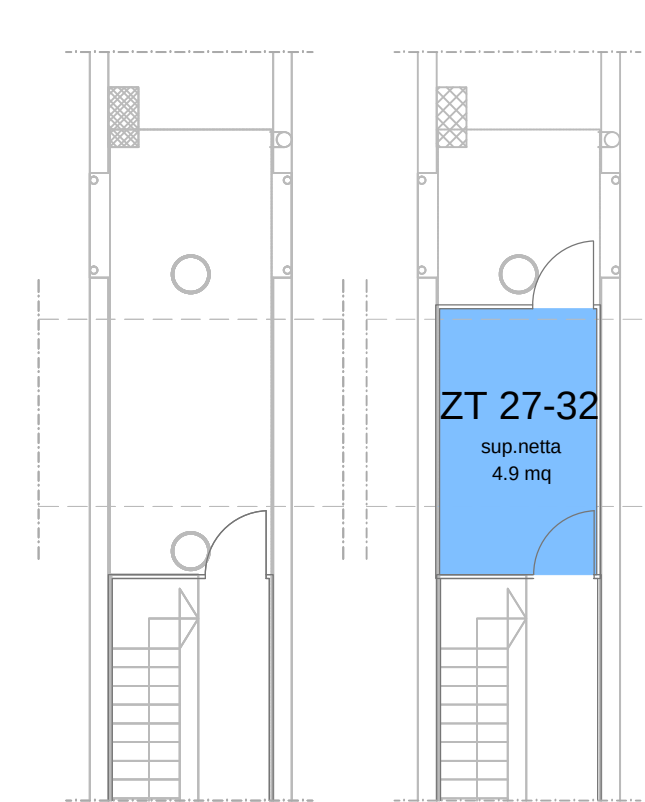
Planta piano terra - cabine di esazione scala 1:150
