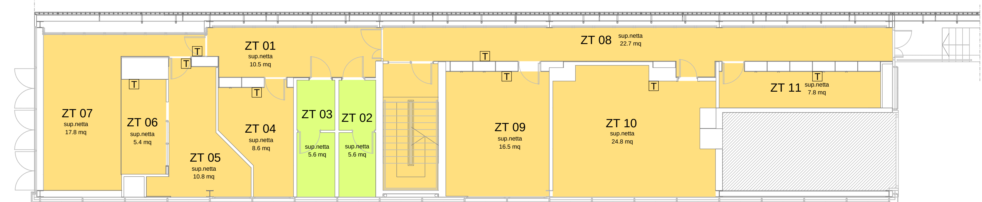
Pianta piano terra - edificio stazione scala 1:150
