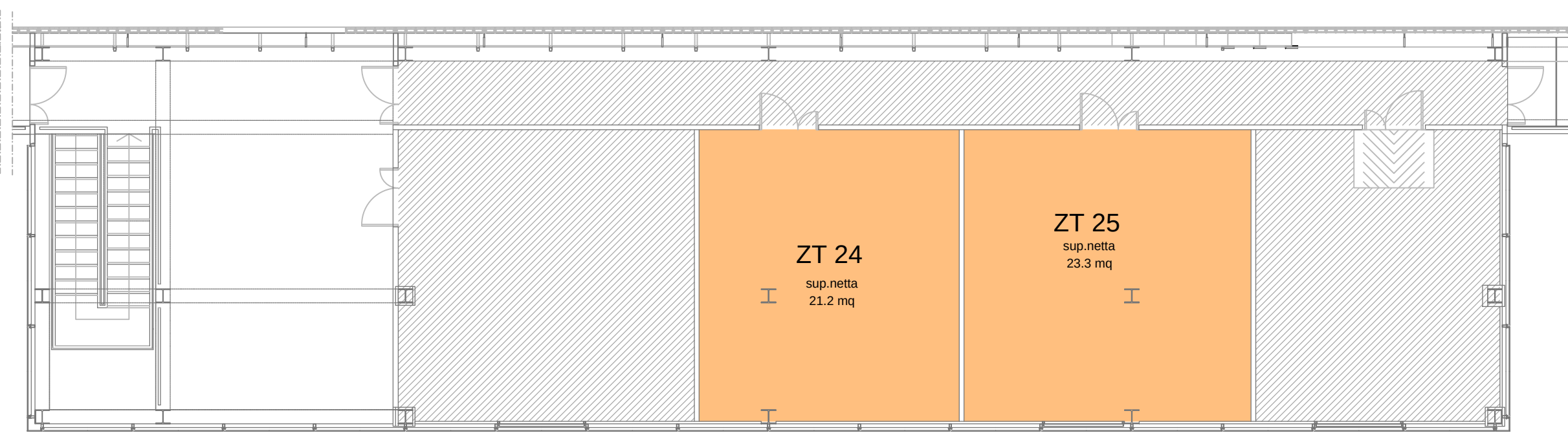
Pianta piano primo - blocco impianti scala 1:150
