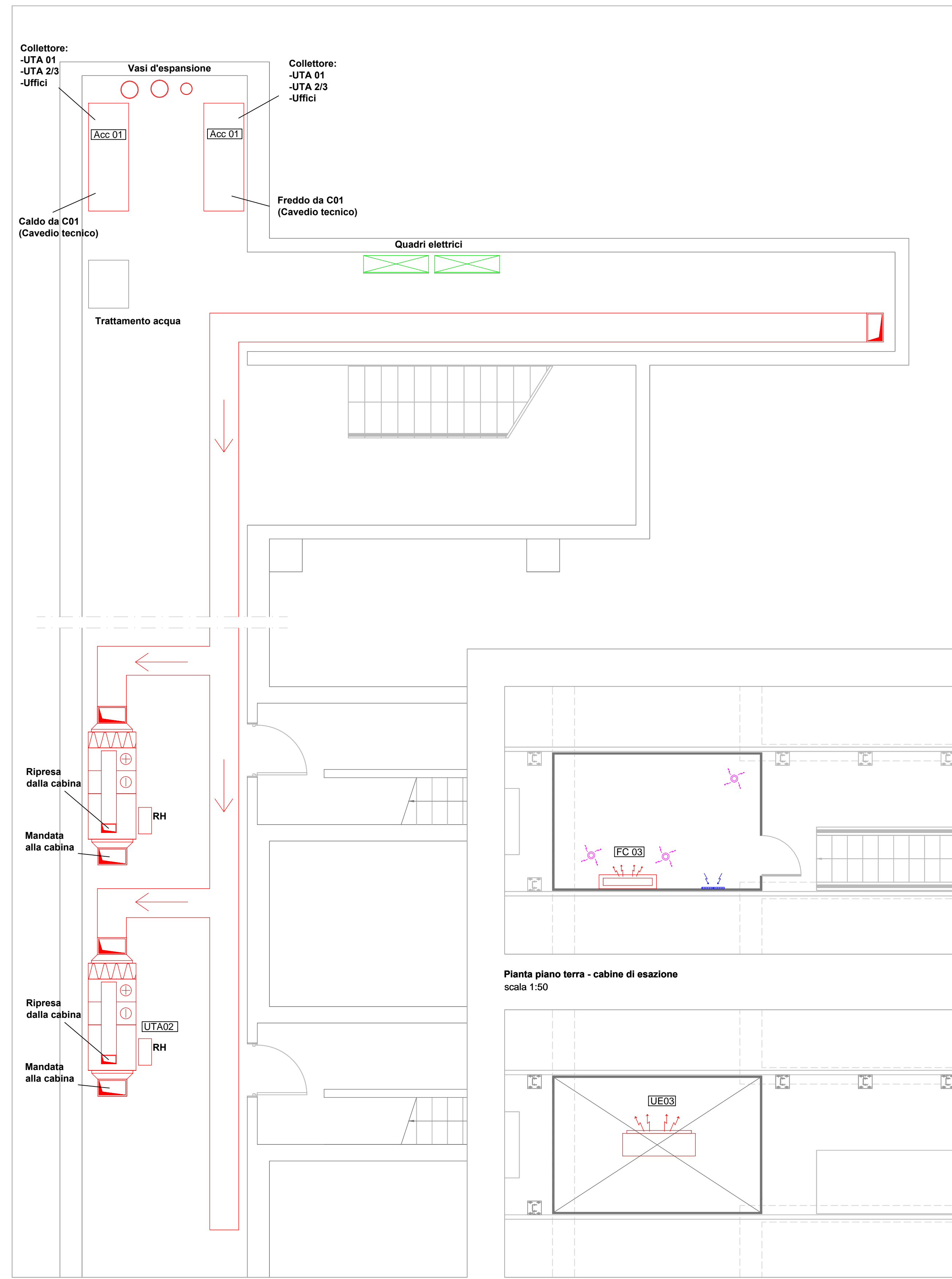
PIANTA PIANO INTERRATO - TUNNEL DI ACCESSO ALLE CABINE DI ESAZIONE scala 1:50
